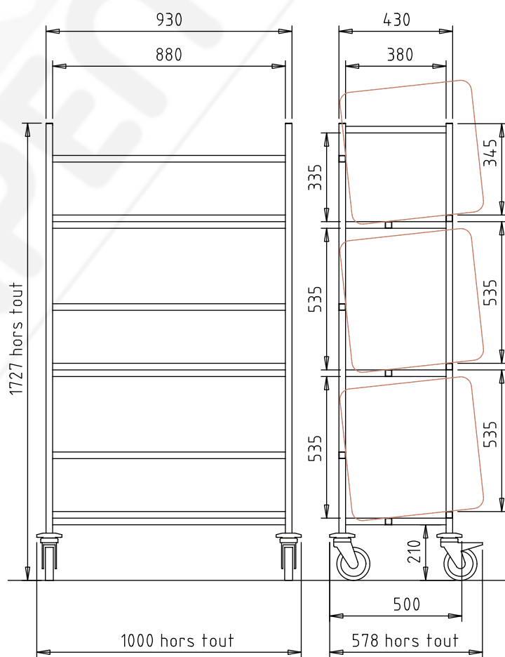
référence 804 196
