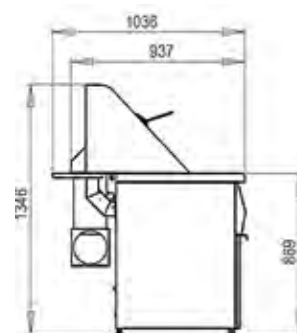
Avec aspiration
