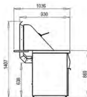
Avec cheminée
