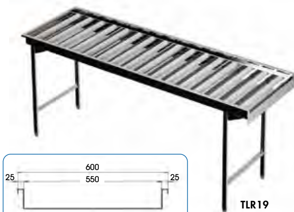
COUPE D'UNE TABLE TLR
