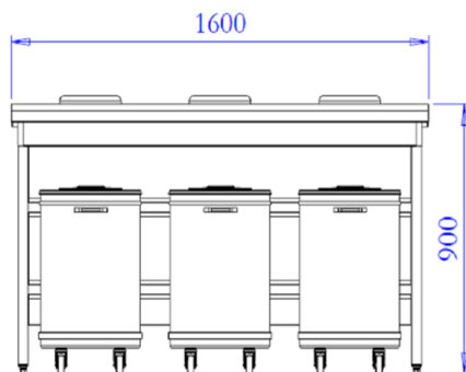
TVP7163P
