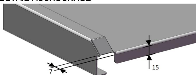
DETAIL ACCROCHAGE
