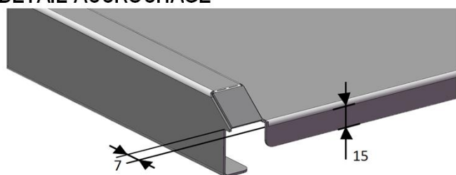
DETAIL ACCROCHAGE
