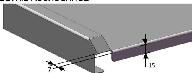
DETAIL ACCROCHAGE
